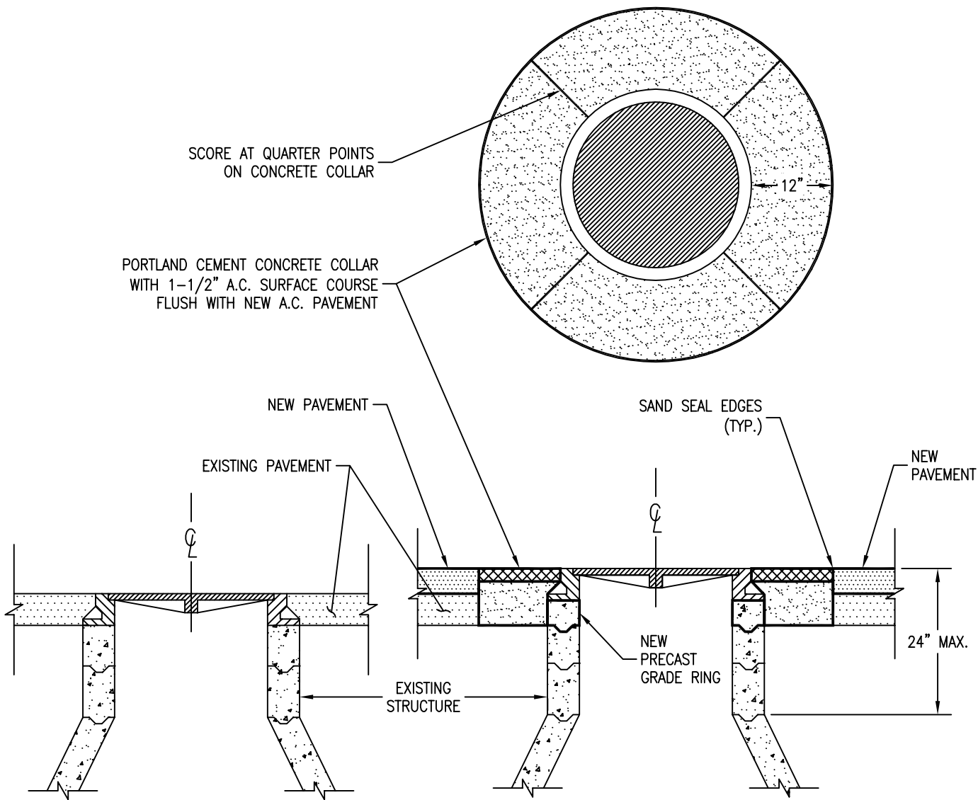
EXISTING MANHOLE NO SCALE
